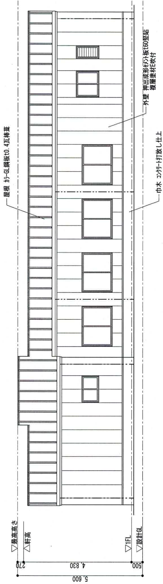
北立面図
